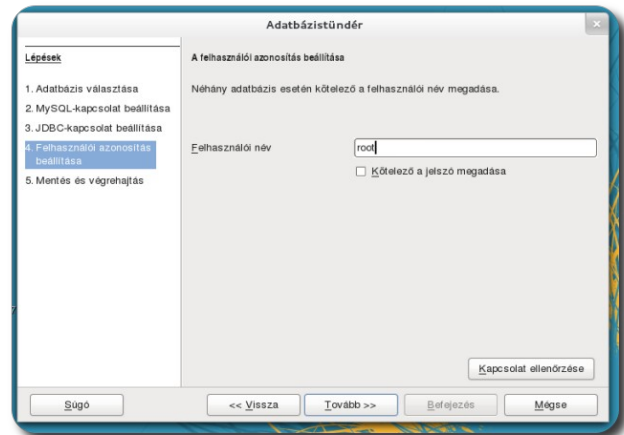
Adatbázis-felhasználó megadása
