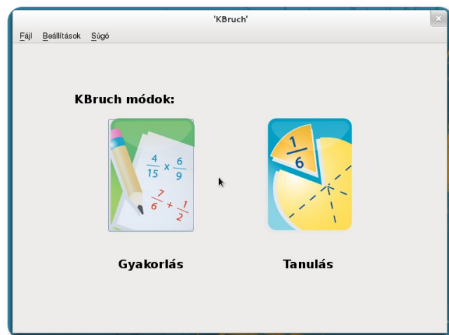
KBruch nyitóképernyője
