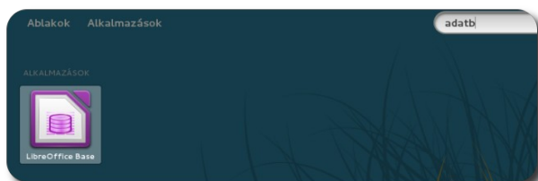
Adatbázis-kezelő indítása
