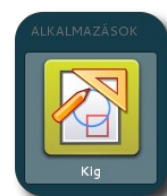
Kig indítása
