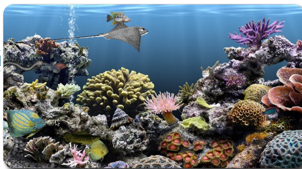
Ügyességi feladat
