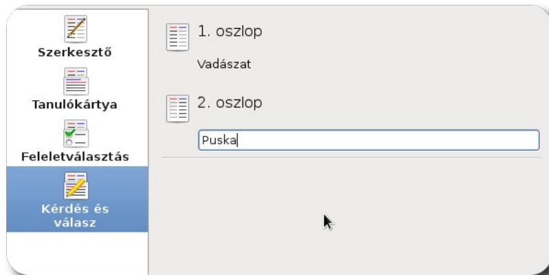
Válasz megadása
